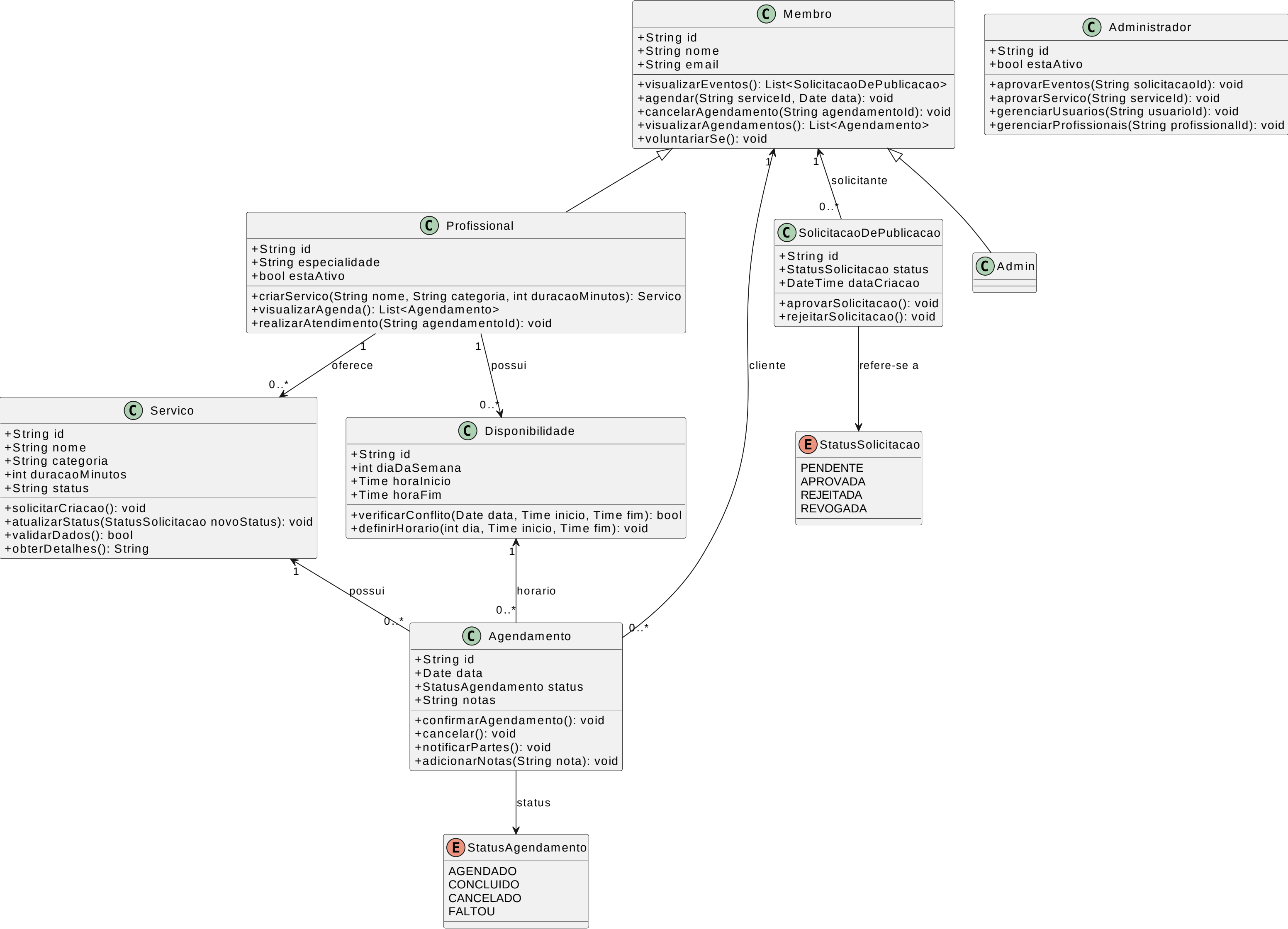
Centro Social App - Diagrama de Classes Consolidado
